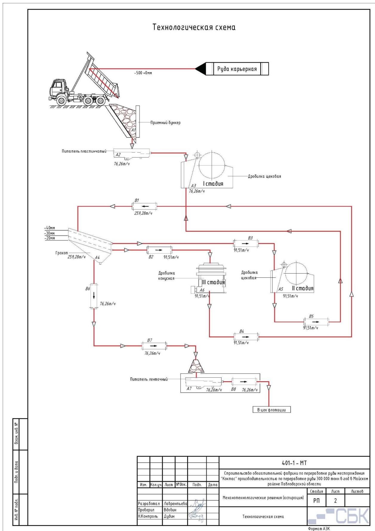
Рисунок 1.6.1 – Технологическая схема ДСК
