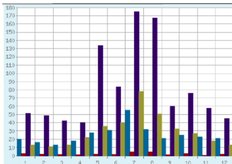
Рисунок 2.4 – Диаграмма осадков по данным таблицы 2.5
