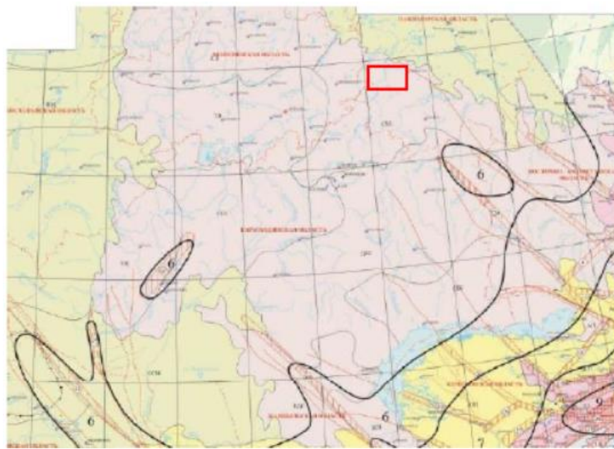
Рисунок 2.6 – Карта районирования территории РК по снеговым нагрузкам
