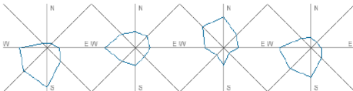
Рисунок 2.2 – Розы ветров.
