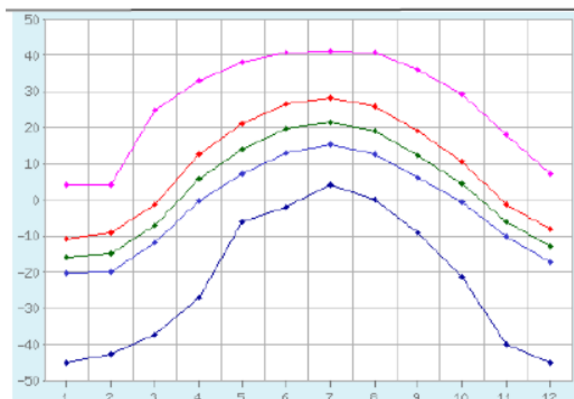
Рисунок 2.1 – Диаграмма температуры воздуха по данным таблицы 2.2
