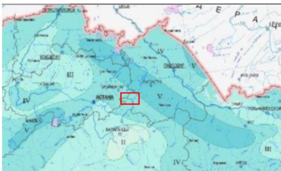
Рисунок 2.3 – Карта районирования территории Павлодарской области по базовой скорости ветра
