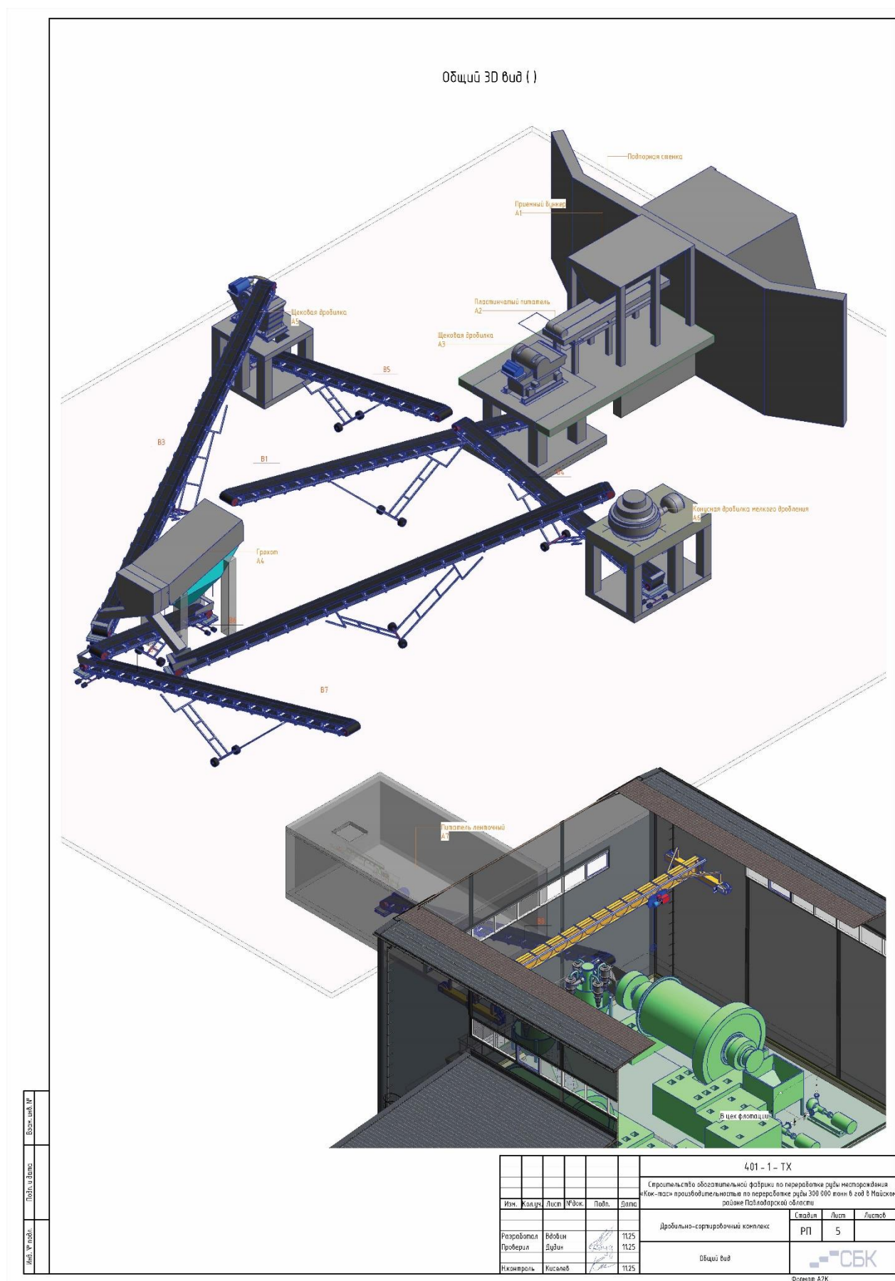
Рисунок 1.6.2 – Технологическая схема ДСК
