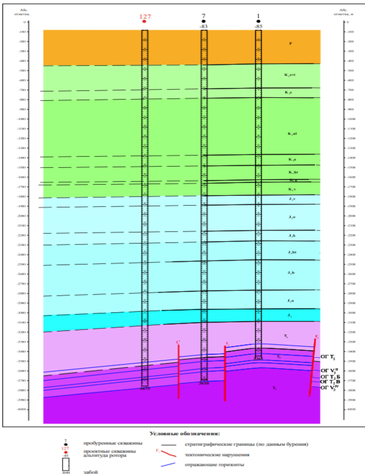
Рисунок 4.3 – Стратиграфический разрез и проектная скважины № 127.
