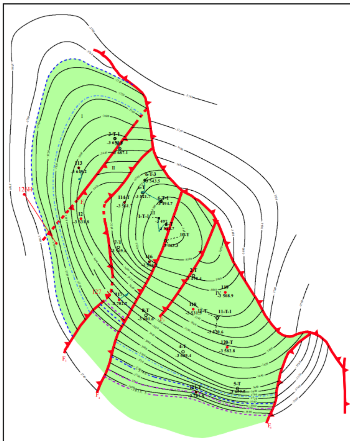
Рисунок 4.2 – Расположения пробуренных и проектная скважины №127 горизонт Т 2 -Б
