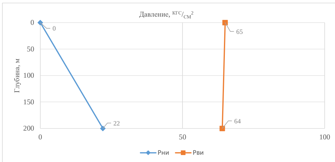
Рисунок 9.1 – Распределение избыточных внутренних и наружных давлений по длине колонны Ø 426 мм (кондуктор)
