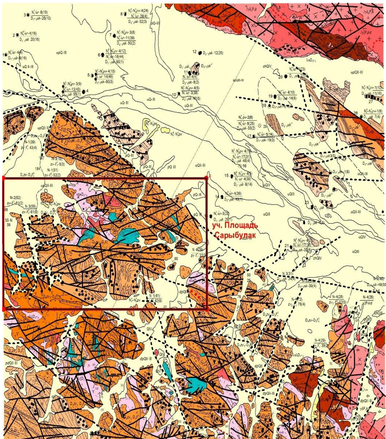
Рисунок 4 - Геологическая карта района работ (М-43-144-Б) (масштаб 1: 50000)
