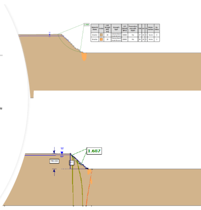
Геотехнический разрез 2502 и 2503
