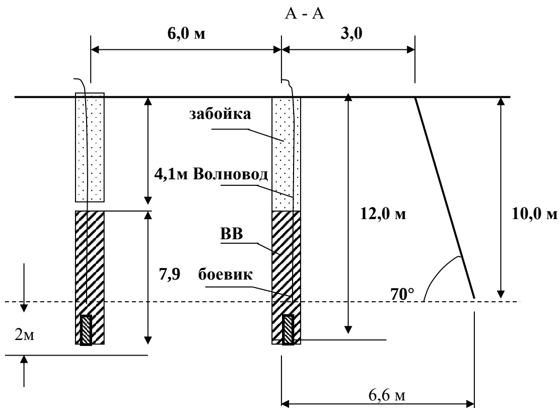
Рис. 5.3 -Конструкция заряда по породе
