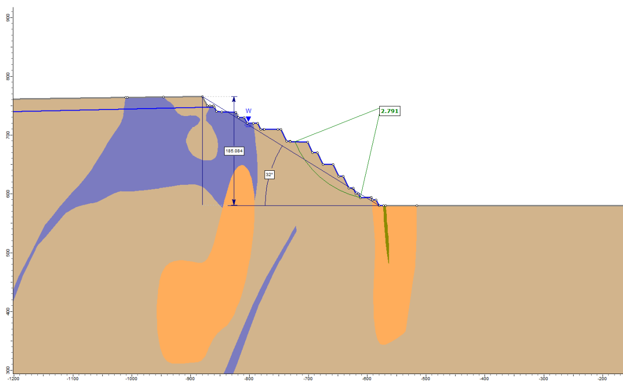
Геотехнический разрез 2507
