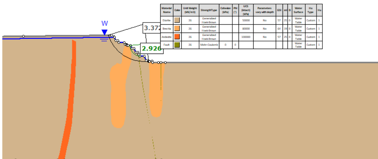
Геотехнический разрез 2511
