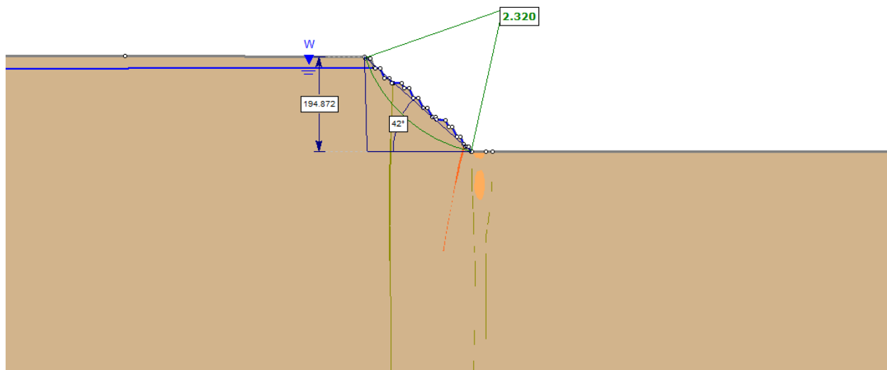
Геотехнический разрез 2506
