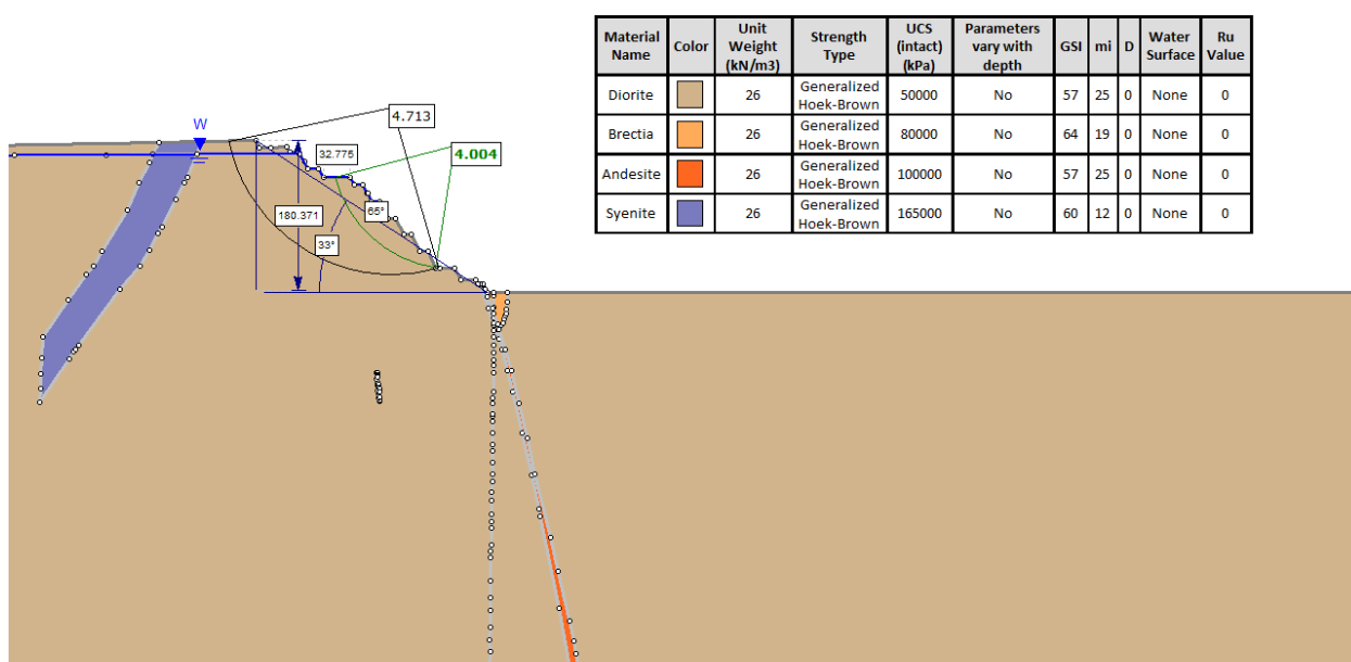
Геотехнический разрез 2505
