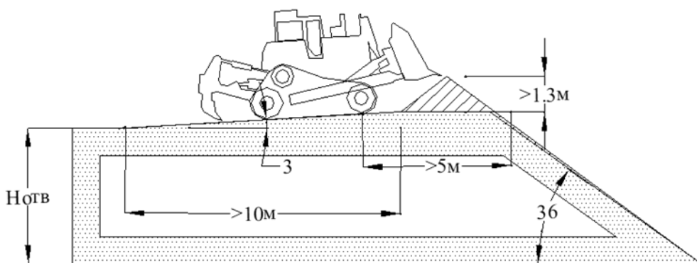
Рисунок 5.15. Формирование разгрузочной площадки отвала бульдозером.
