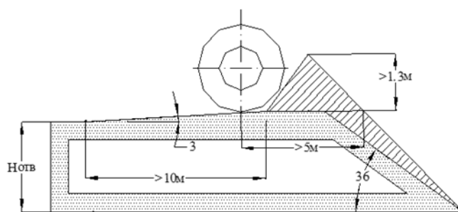
Рисунок 5.14. Схема разгрузочной площадки отвала
