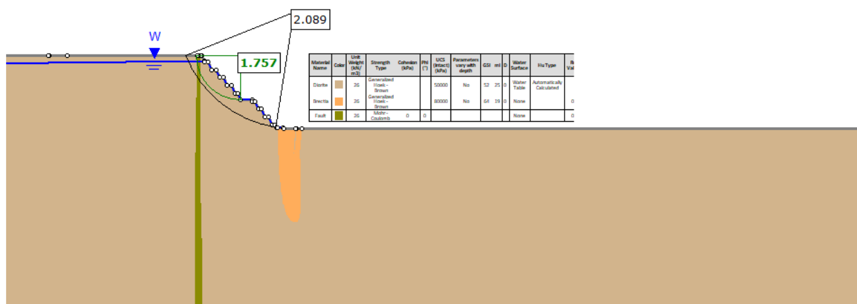
Геотехнический разрез 2508
