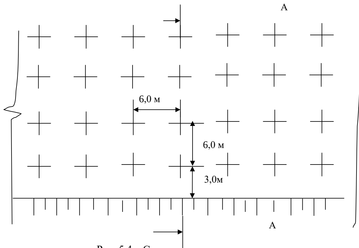
Рис. 5.4 – Схема расположения скважин по породе
