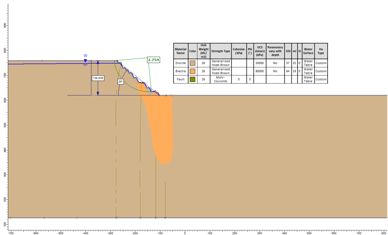
Геотехнический разрез 2513
