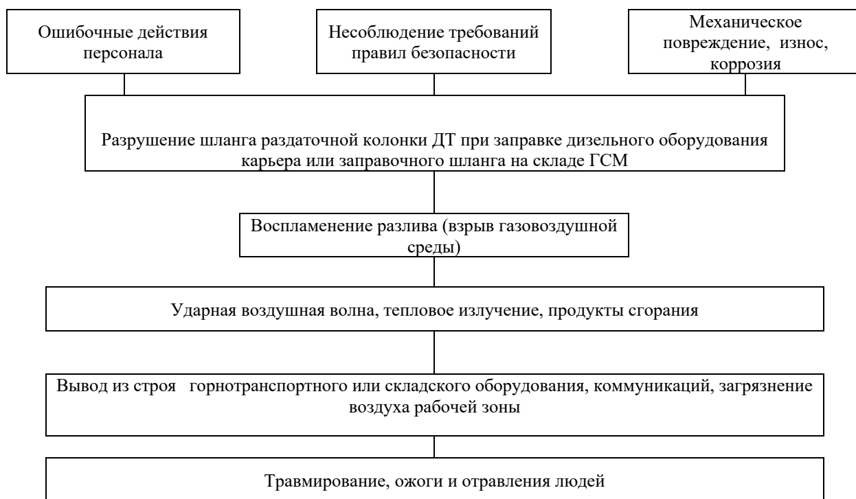
Рисунок 8.3 - Блок-схема вероятного сценария возникновения и развития аварии при заправке дизельного технологического оборудования карьера из топливозаправщика или заправке емкости на складе ГСМ
