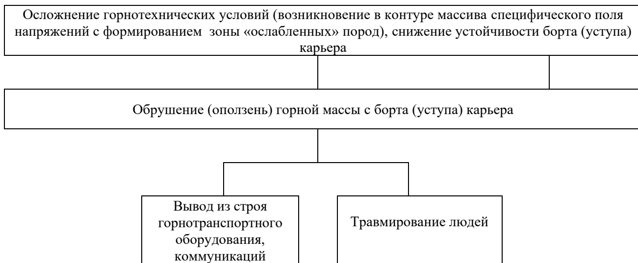
Рисунок 8.1 - Блок-схема вероятного сценария аварии при обрушении (оползней) горной массы с борта (уступа) карьера
