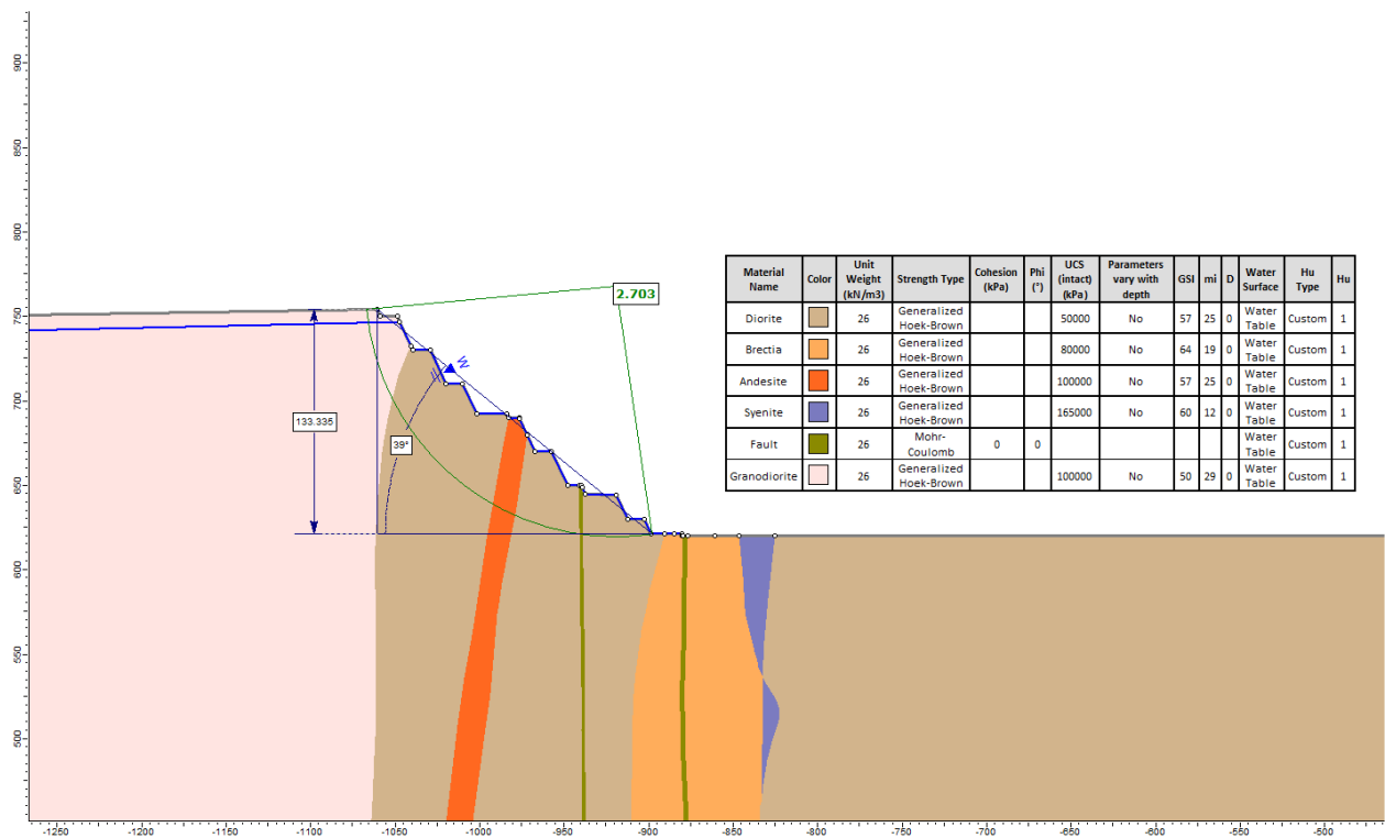
Геотехнический разрез 2512
