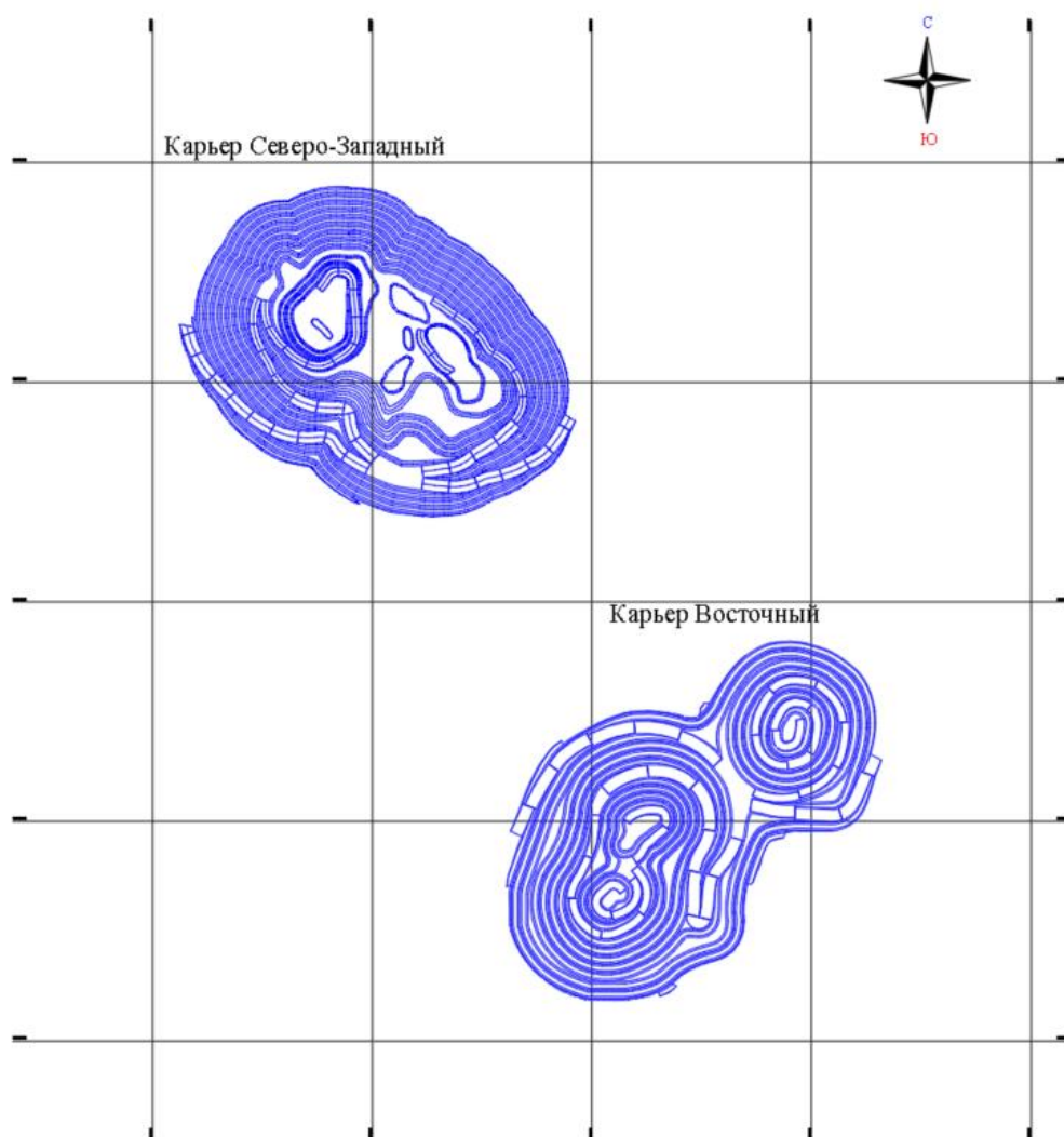
Рис. 5.2 Проект карьеров Восточный и Северо-Западный.
