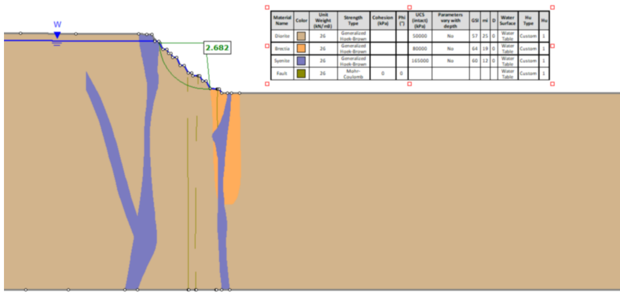
Геотехнический разрез 2510
