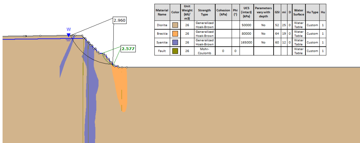
Геотехнический разрез 2509
