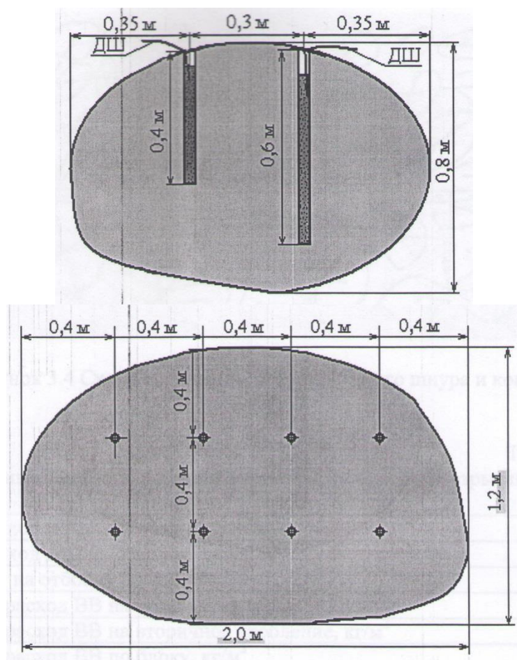
Рис. 3.3 Конструкция заряда при вторичном дроблении
