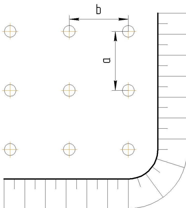
Рис. 2.5 – Типовые элементы расположения скважин и расчет зарядов
