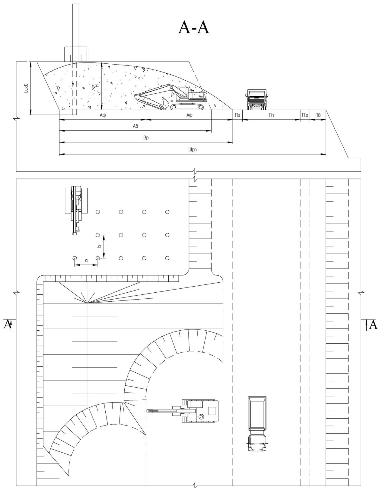
Рис. 2.3 - Параметры рабочей площадки при отработке уступа (подступа) экскаватором с погрузкой в автосамосвал.
