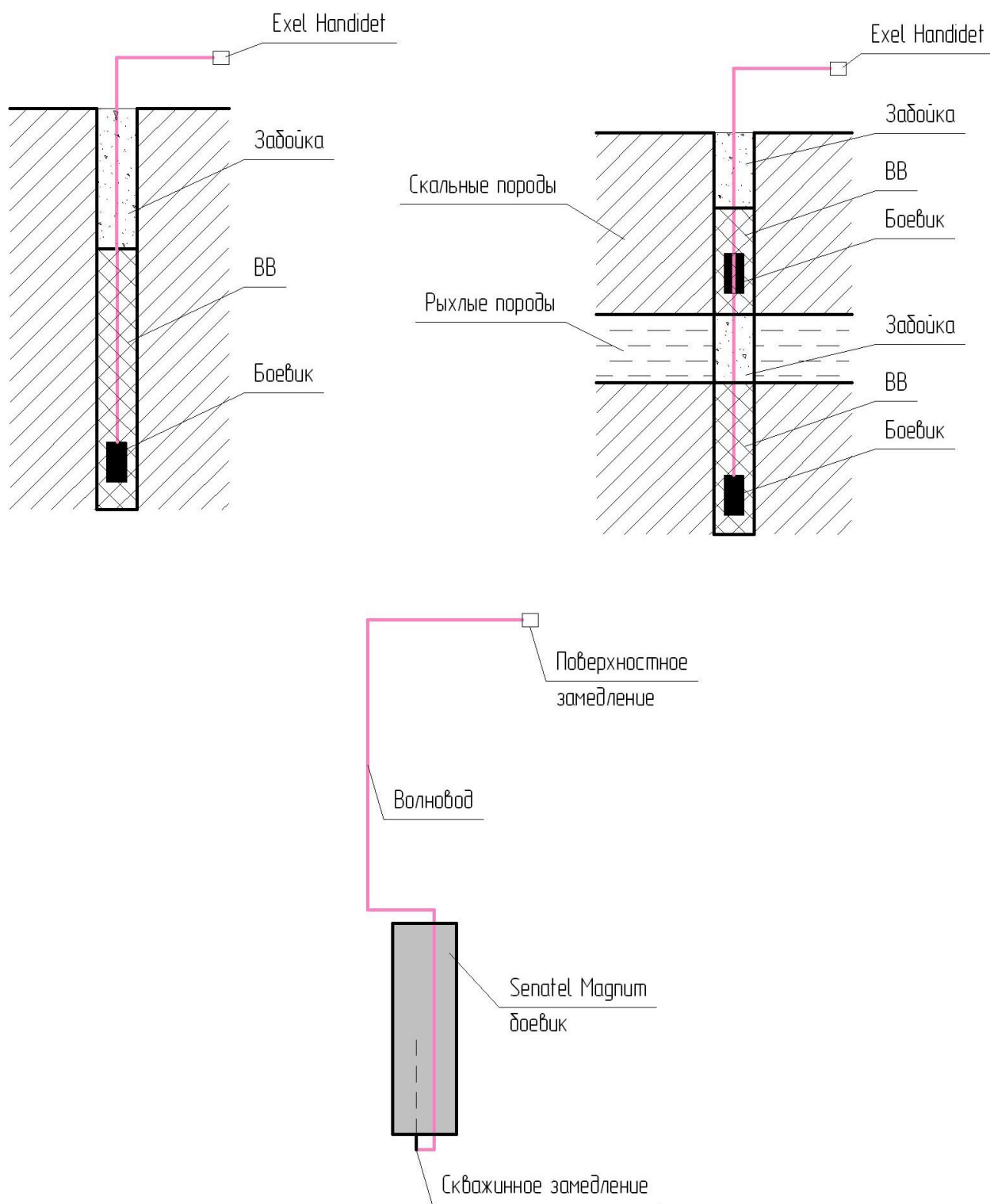
Рис. 2.8 – Конструкция заряда
