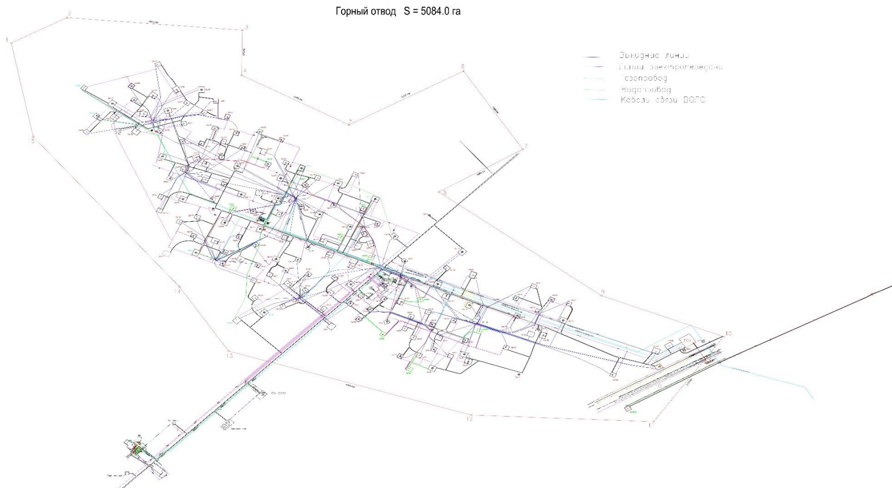
Рисунок 2 – Схема расположения производственных площадок
