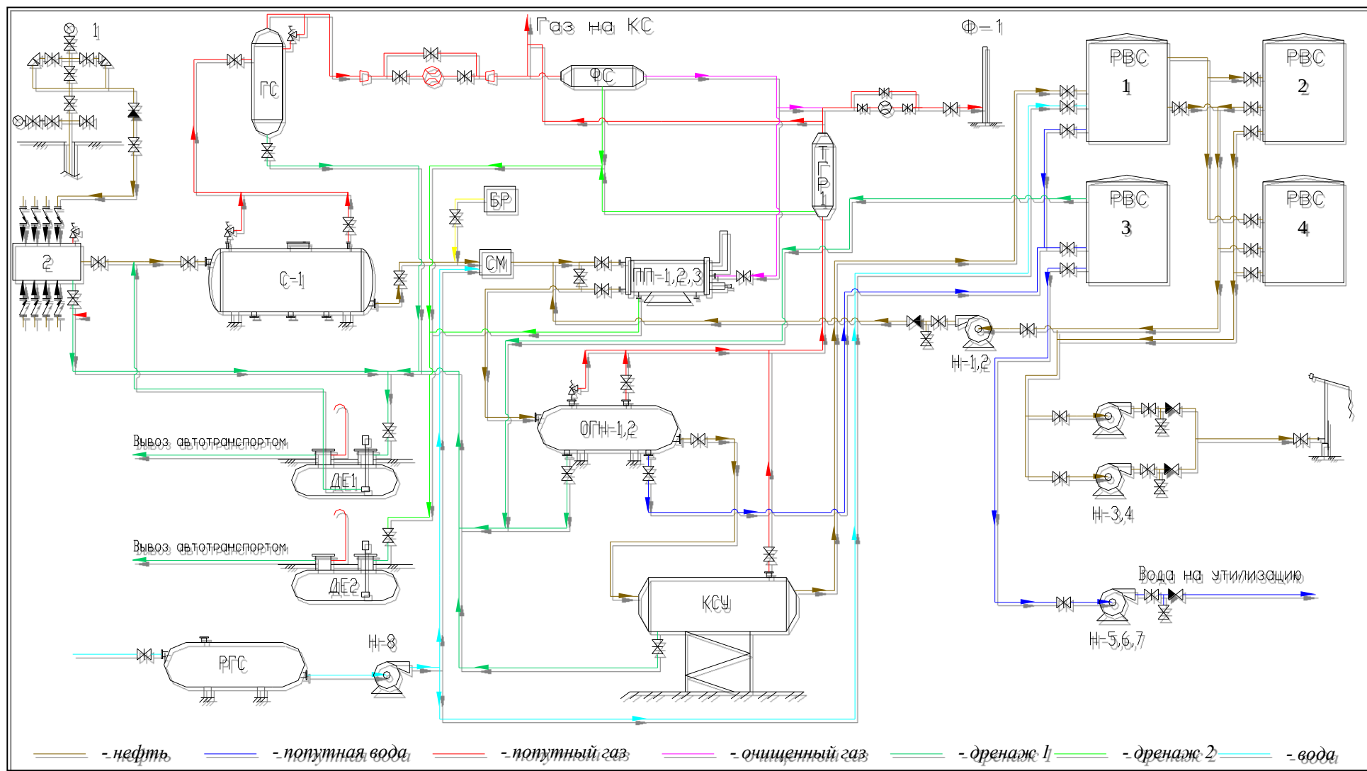
Рисунок 3 – Принципиальная технологическая схема УПП
