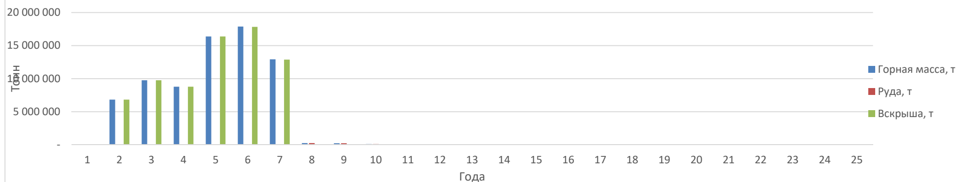
Рисунок 2.4 – Сводный график режима горных работ (участок 19.9)
