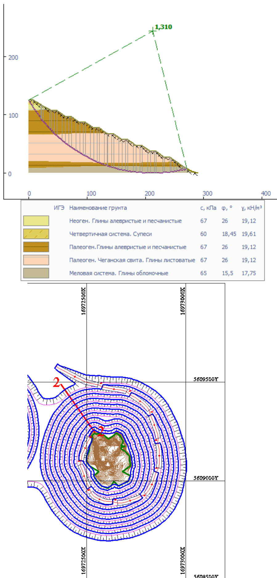
Рисунок 2.1 - Геологический разрез по карьере 19.6
