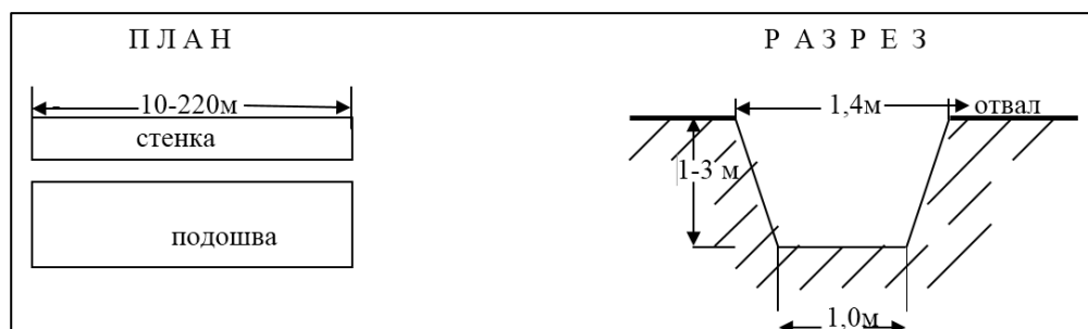
Рисунок 5. Паспорт проходки канав глубиной до 2 м
