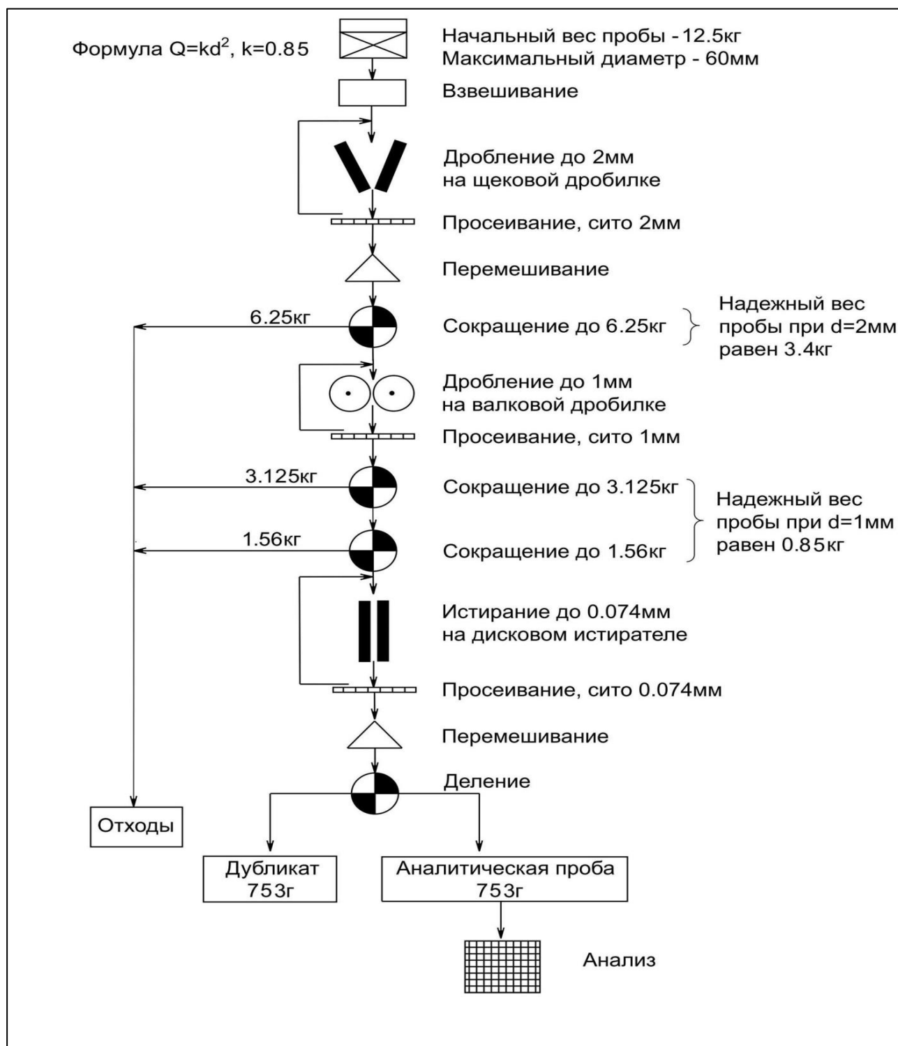
Рисунок 6. Схема обработки бороздовых проб
