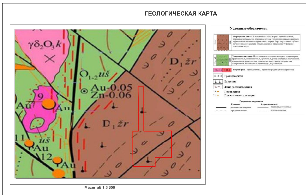
Рисунок 3. Геологическая карта района работ Перспективный-3
