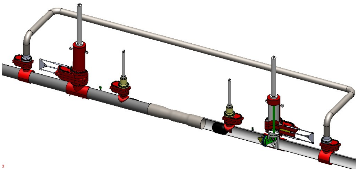
(Рисунок 5) Установка устройства для перекрытия (тампонажного пакера), выполнение работ по перекрытию
