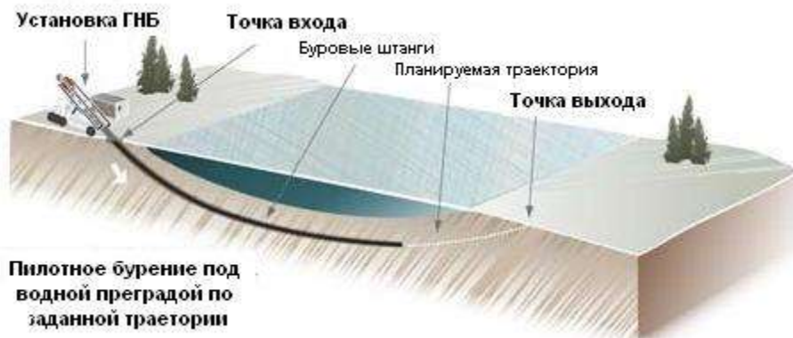
Рисунок 1.5.1 – Наклонно-направленное бурение
