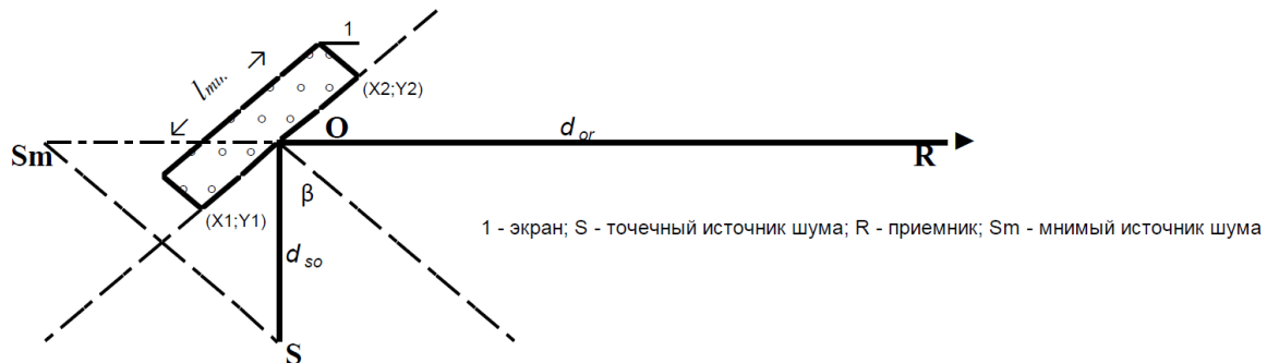
Рисунок 2 - Зеркальное звукоотражение от экрана
