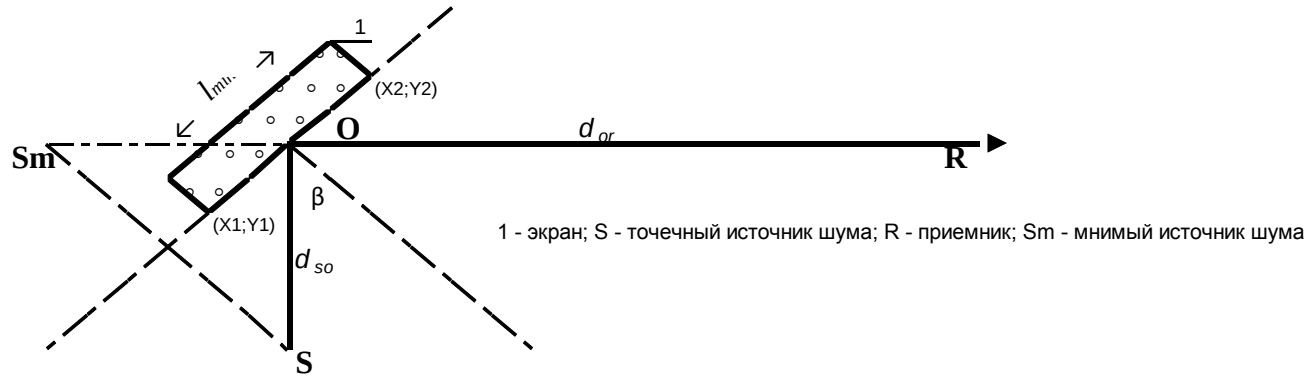
Рисунок 2 - Зеркальное звукоотражение от экрана
