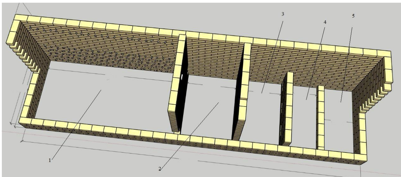
Рисунок 4.2 – Схема Деструктивного инсинератора ZENDA T-100
