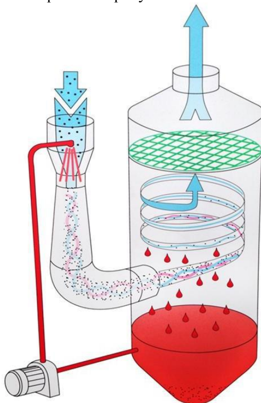
Рисунок 4.3 – Принцип работы Скруббера Вентури Ергоп 1
