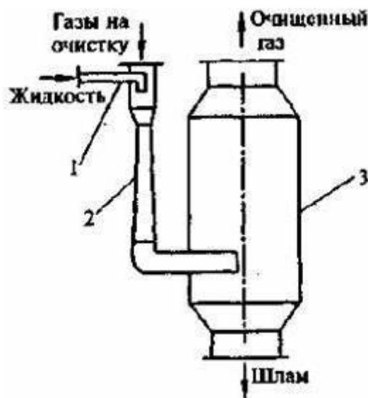
Рисунок 4.4 – Конструкция Скруббера Вентури Еprom 1 1 – орошающая форсунка; 2 – труба Вентури; 3 – каплеуловитель.
