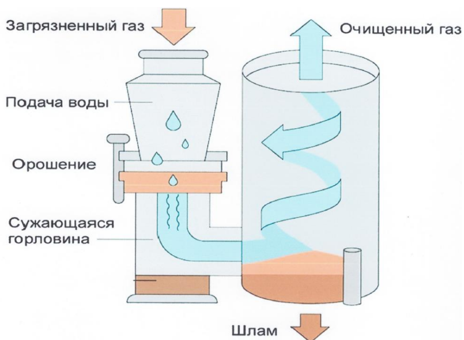
Рисунок 4.5 – Принцип работы Скруббера Вентури SCR-0.1
