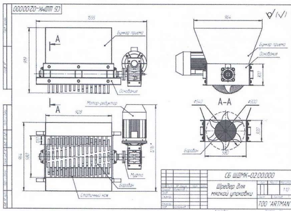
Рис. 2 – Общий вид шредера
