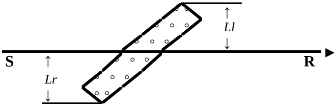
Рисунок 1 - Вид сверху на экран между источником шума S и приемником R
