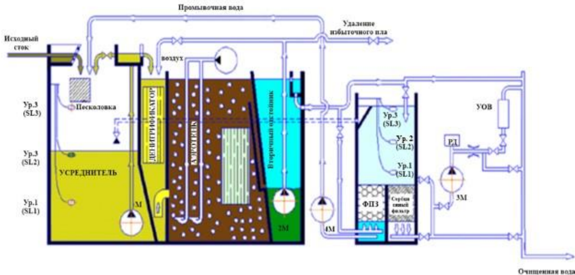
Рисунок 3.5.1 Схема установки биологической очистки сточных вод
