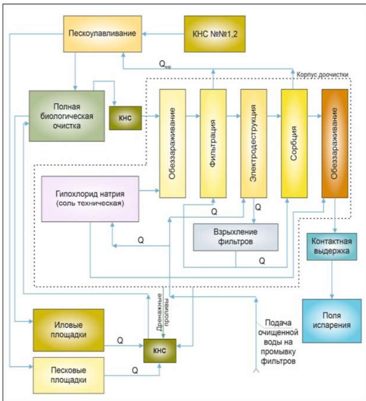
Рисунок 11 - Технологическая схема работы очистных сооружений «Эйкос», производительностью 1500 м 3 /сут
