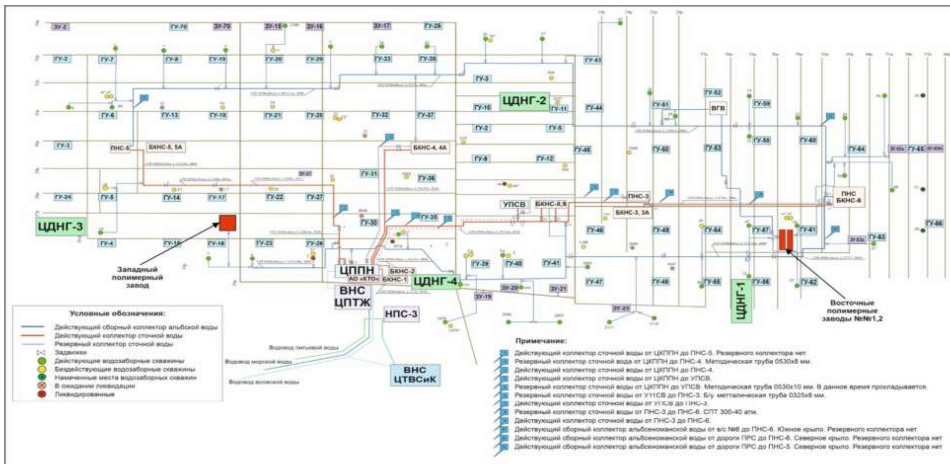
Рисунок 8 - Схема расположения водозаборных скважин и водовода альбсеноманской воды
