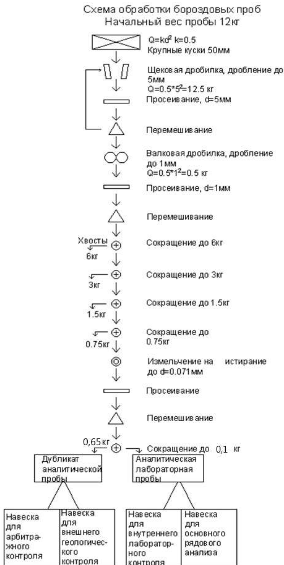
Рис. 5 Схема обработки бороздовых проб 12 кг
