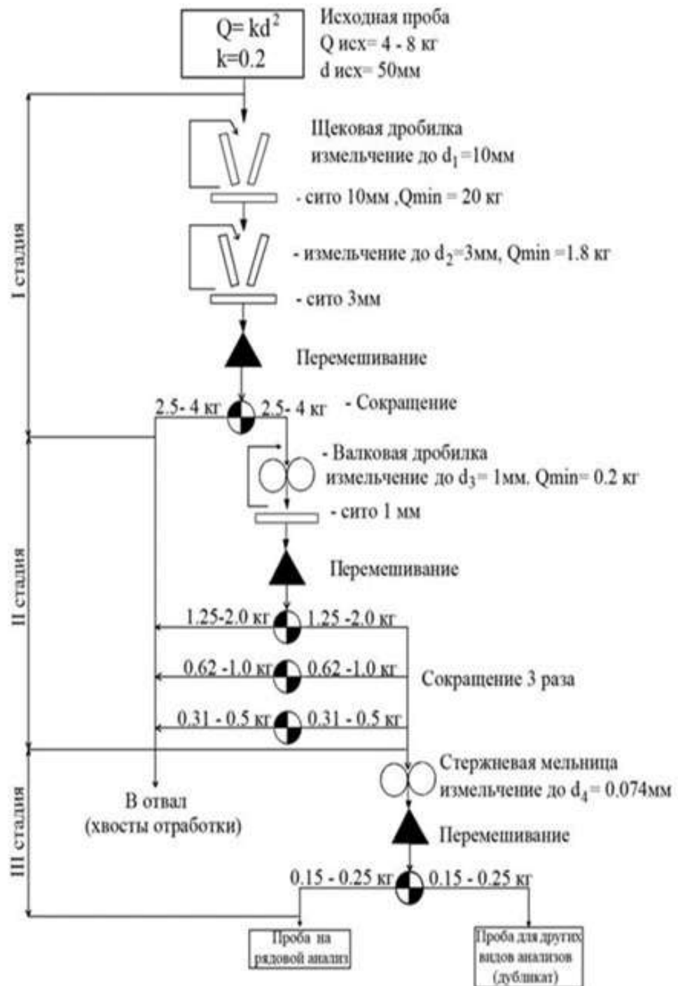
Рис. 6 Схема обработки керновых проб
