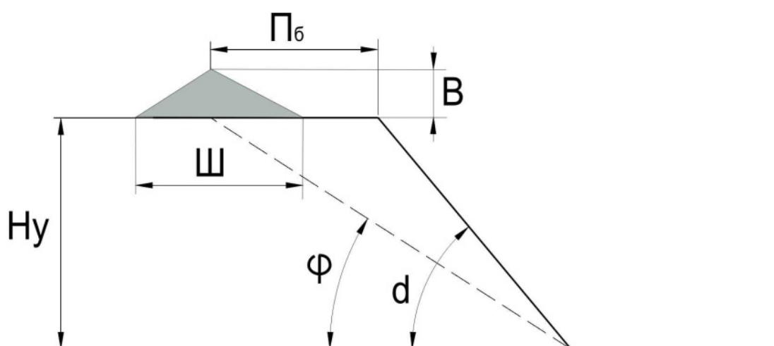
Рис.3.4.1 Схема уступа
