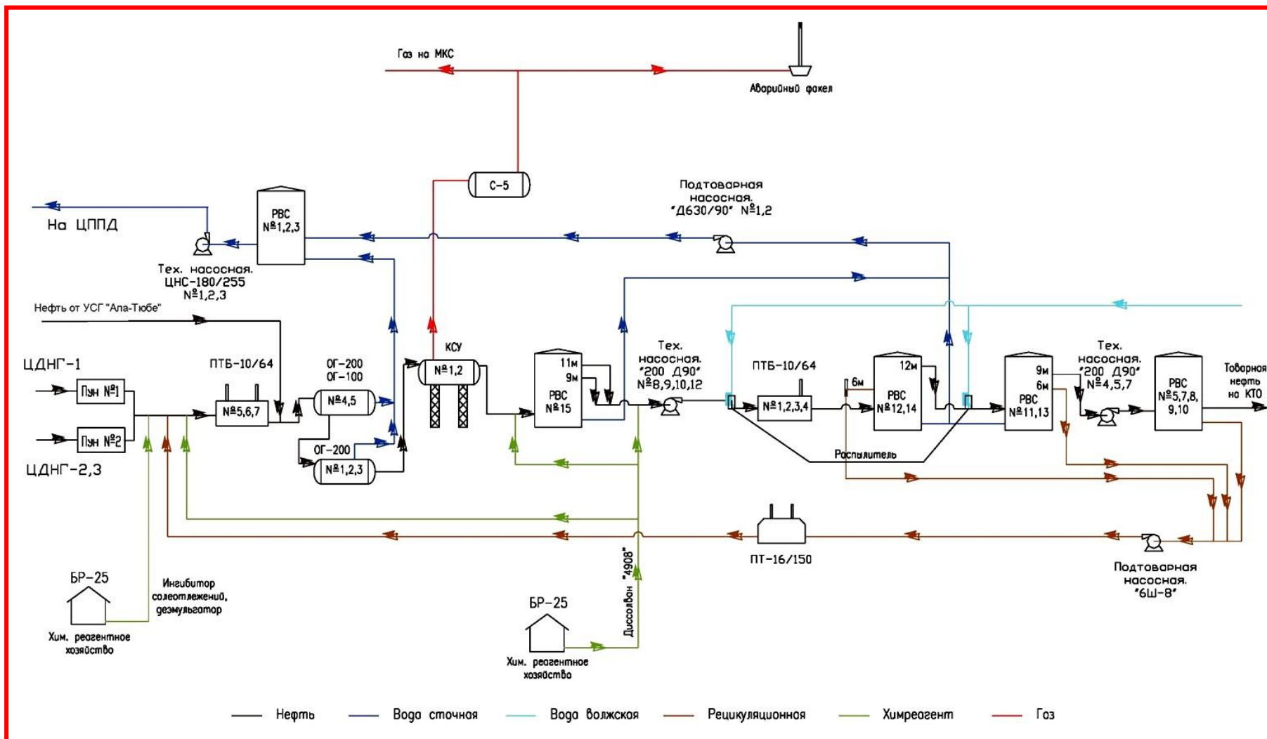
Рисунок 6.2.6. – Технологическая схема подготовки нефти на ЦППН
