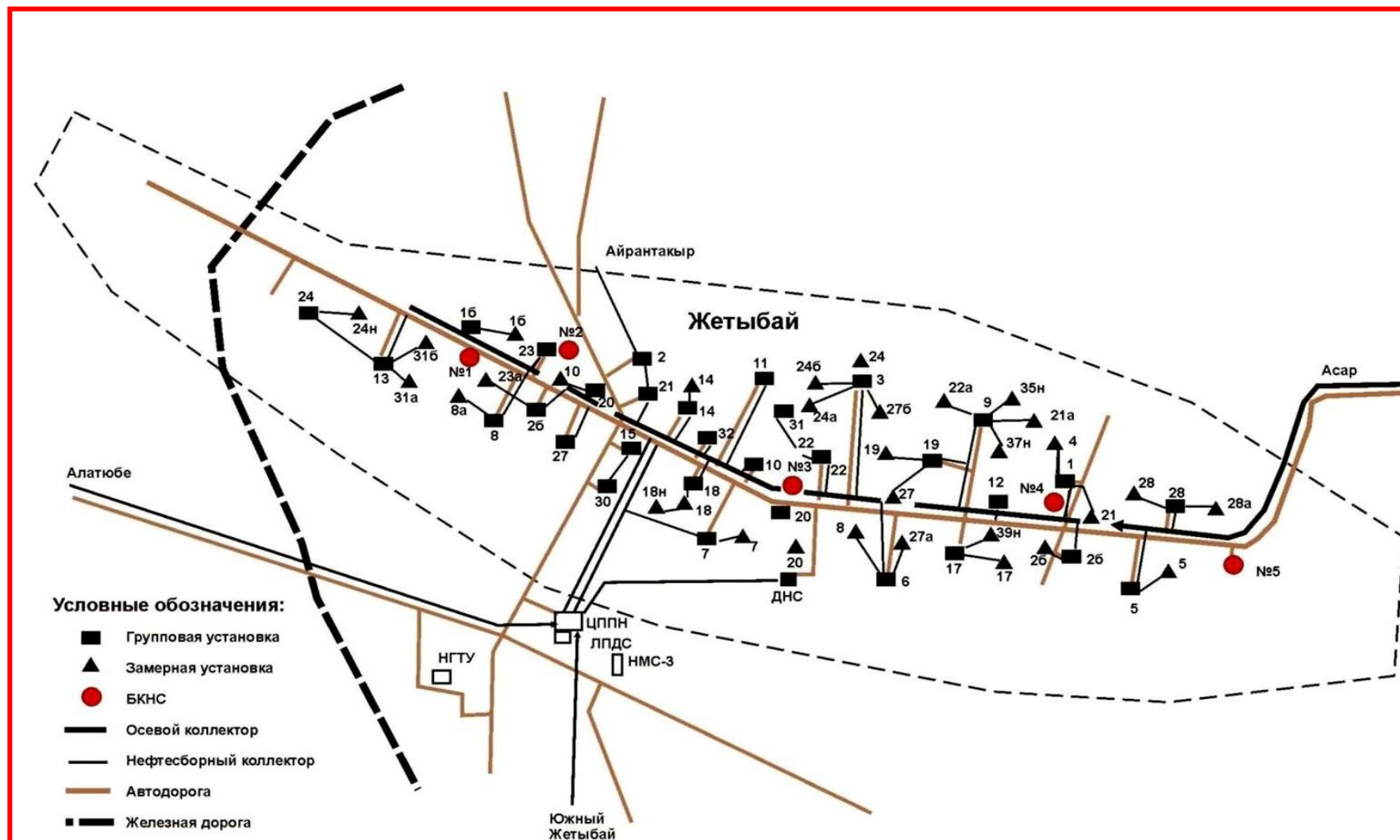
Рисунок 6.2.5 - Принципиальная схема нефтесбора на месторождении Жетыбай
