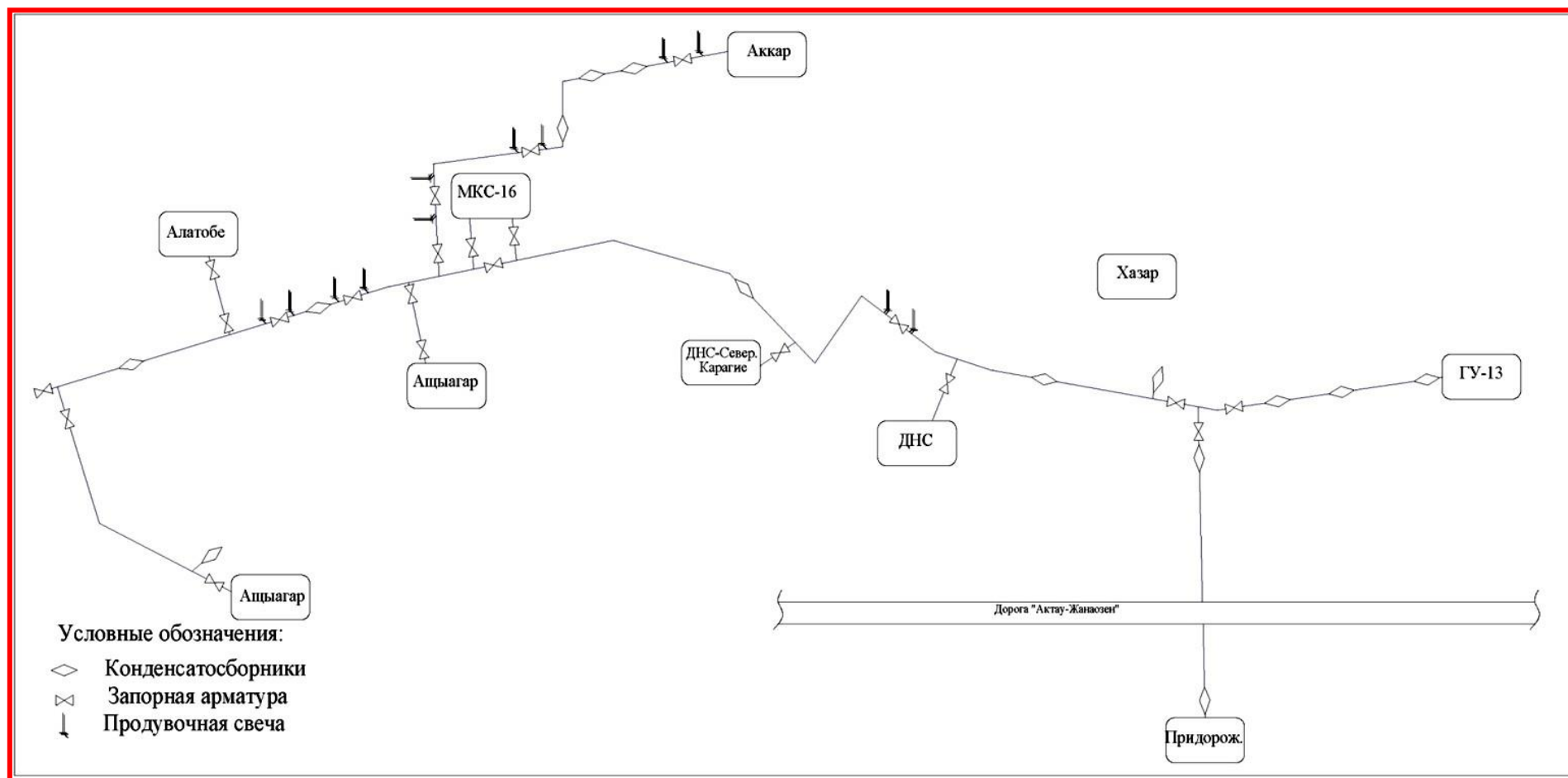
Рисунок 6.2.3 - Схема системы сбора газа малых месторождений ЦДНГ-1
