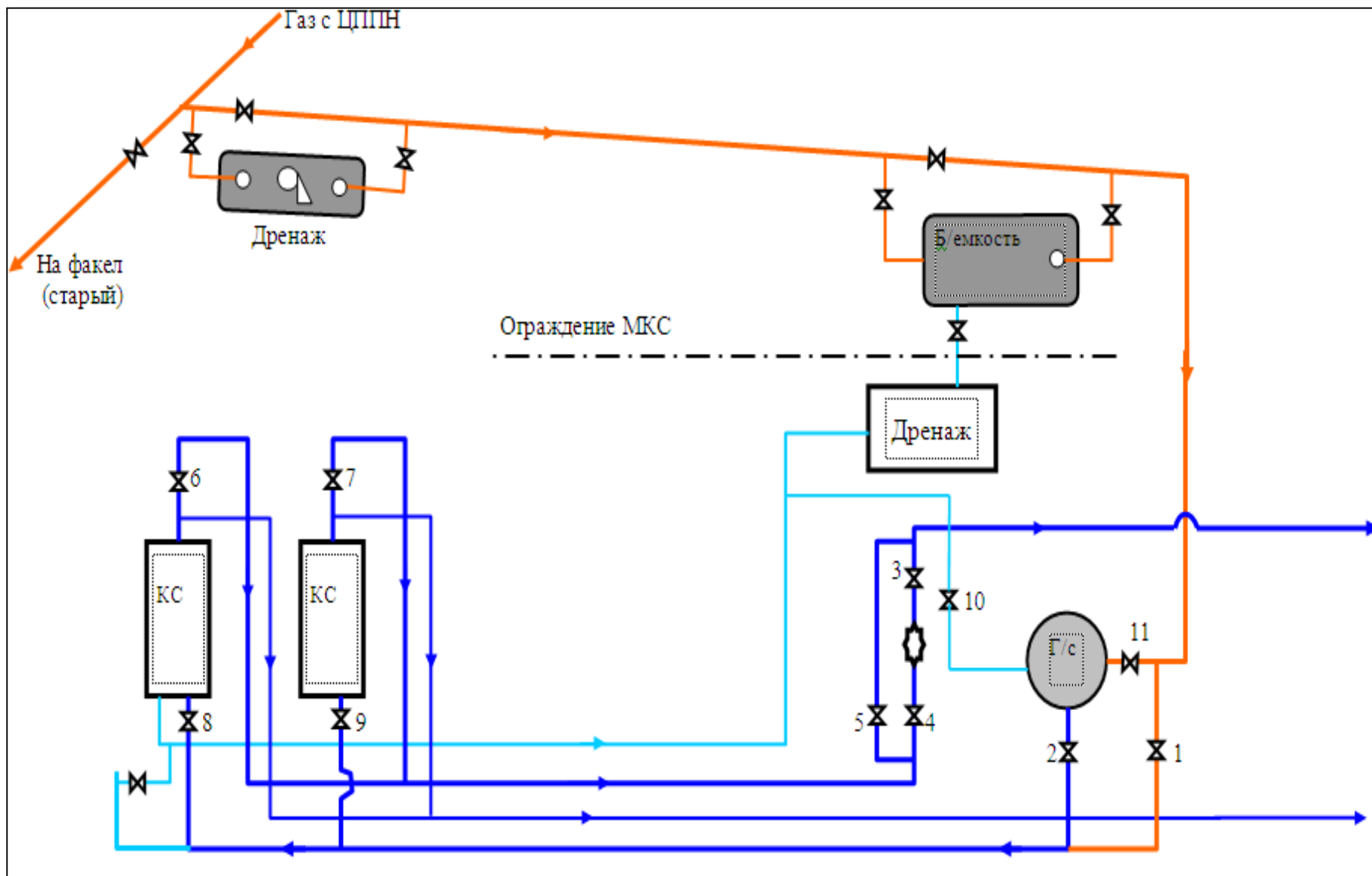
Рисунок 6.2.8. - Принципиальная технологическая схема МКС-13 ЦППН
