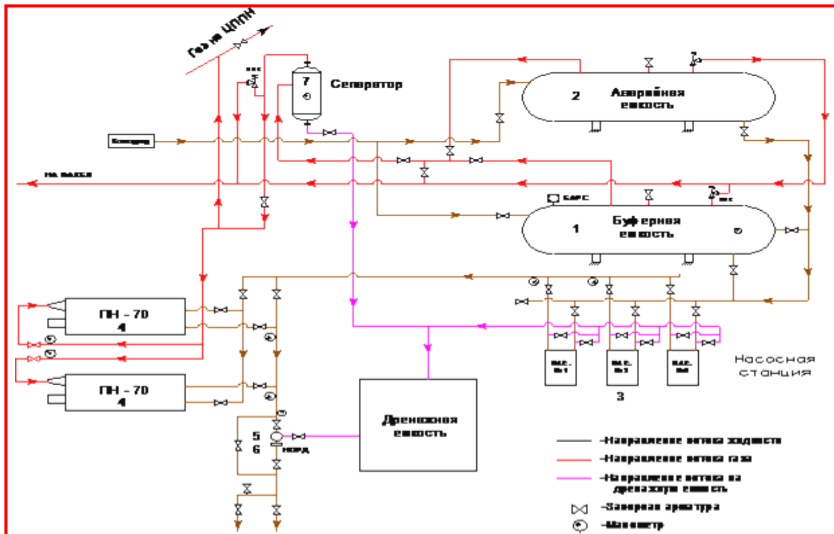
Рисунок 6.2.1.- Технологическая схема ДНС на месторождении Жетыбай
