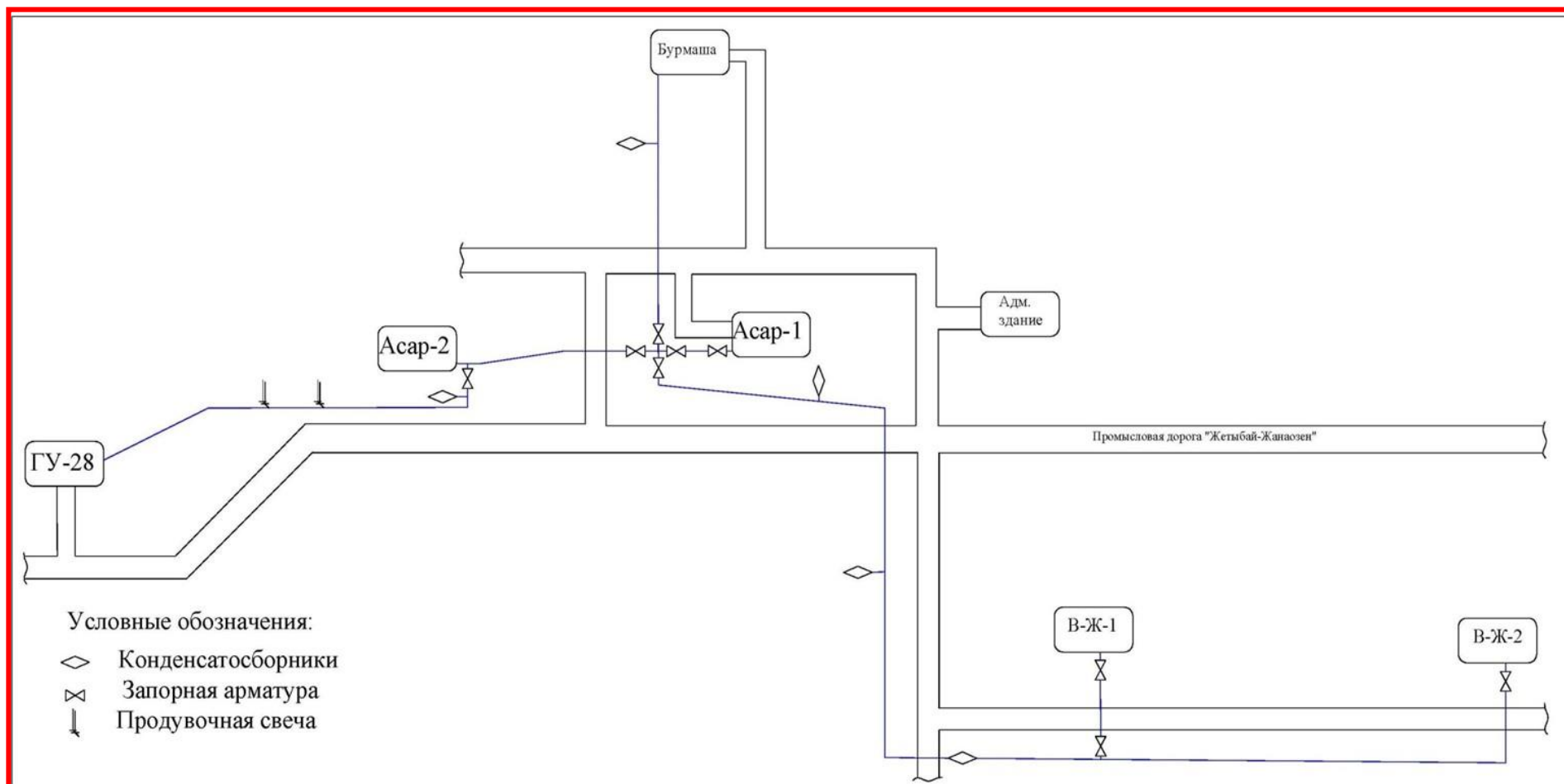
Рисунок 6.2.4- Схема системы сбора газа малых месторождений ЦДНГ-3
