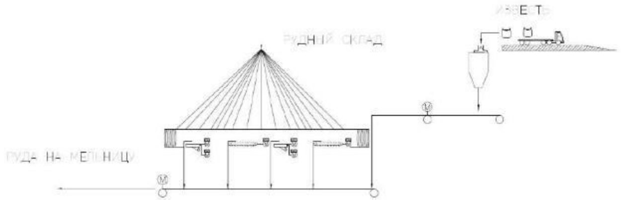
Рисунок 1.8 Схема цепи аппаратов склада руды и подачи извести.
