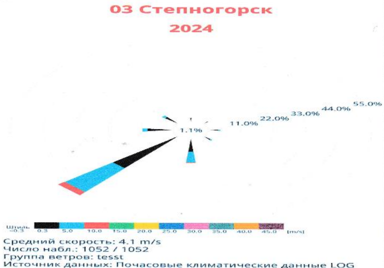
Рисунок 1.6 Среднегодовая роза ветров, %
