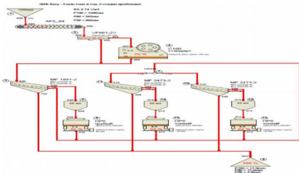
Рисунок 1.7 Схема технологического процесса дробления руды открытой добычи
