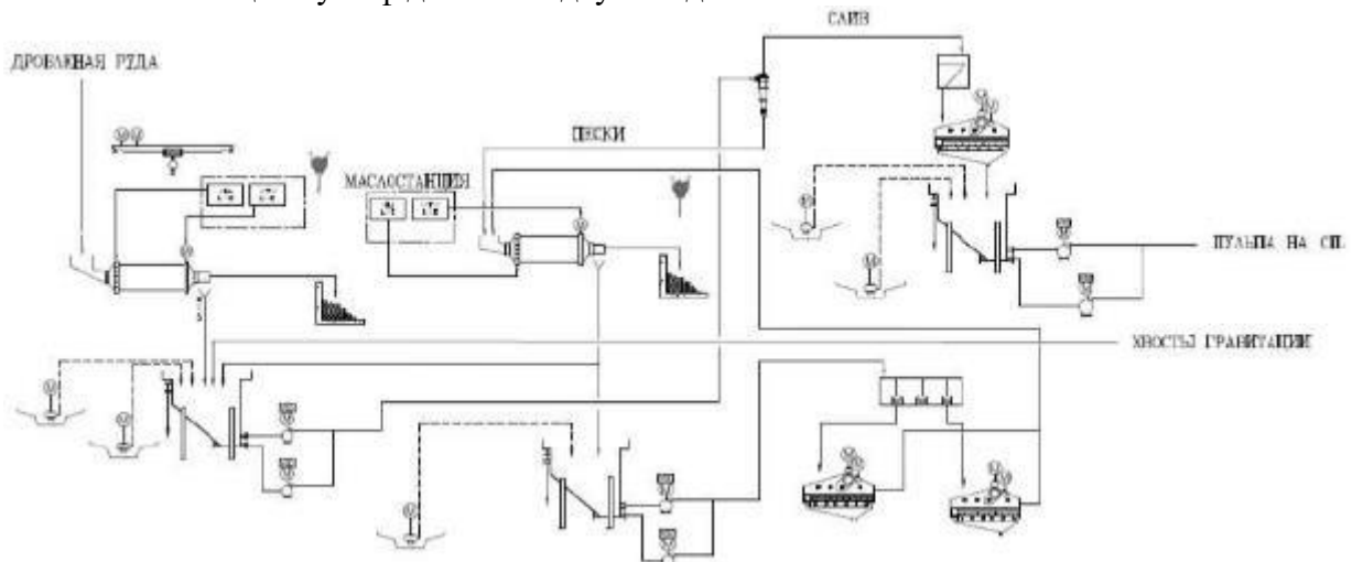
Рисунок 1.9 Схема цепи аппаратов отделения измельчения и классификации.
