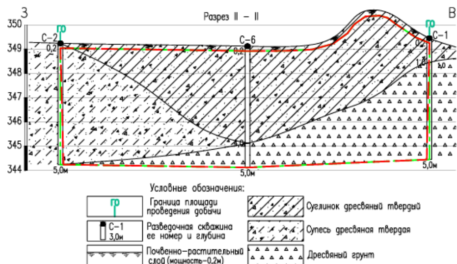
Рис. 2.15. Схема геологического строения участка «№4Ж».
