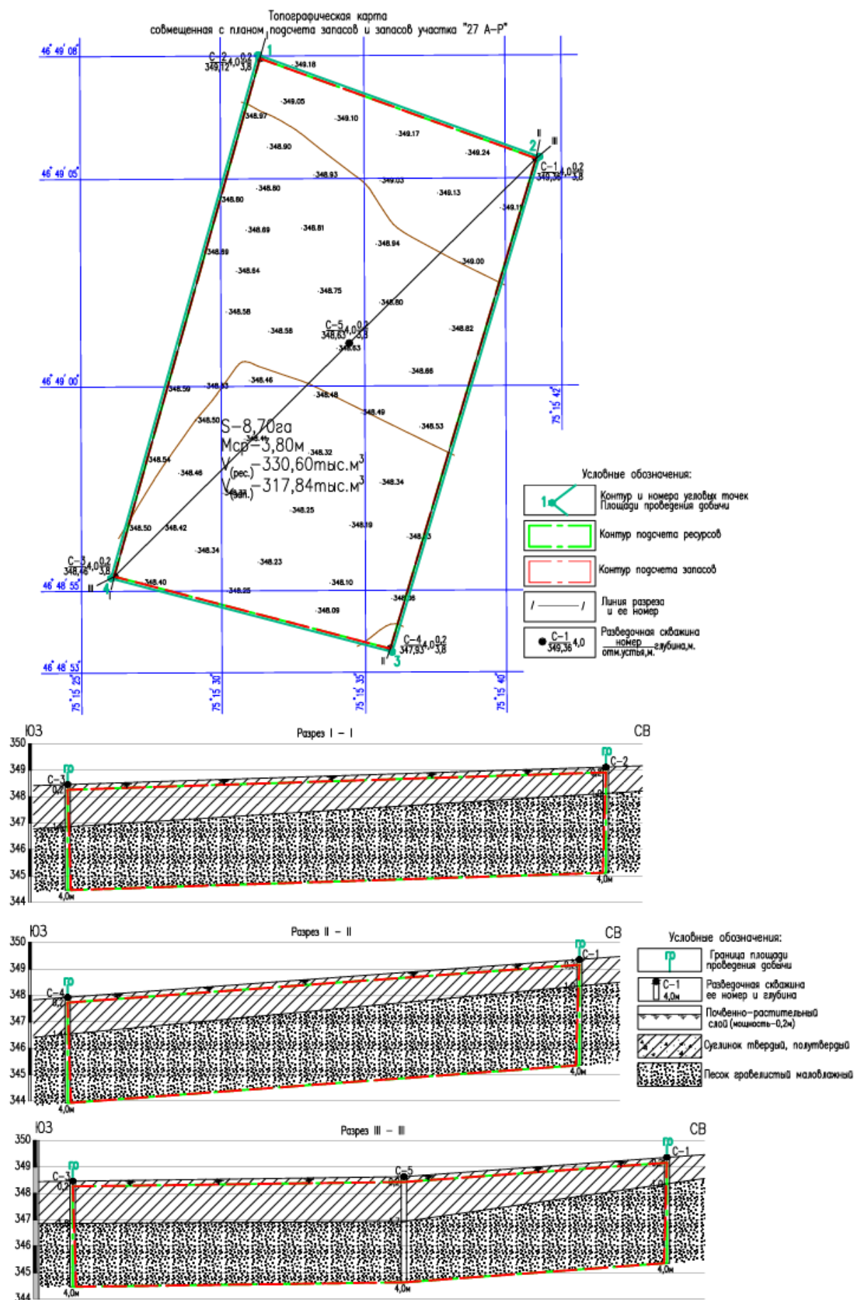
Рис. 2.10. Схема геологического строения участка «№27А-Р».
