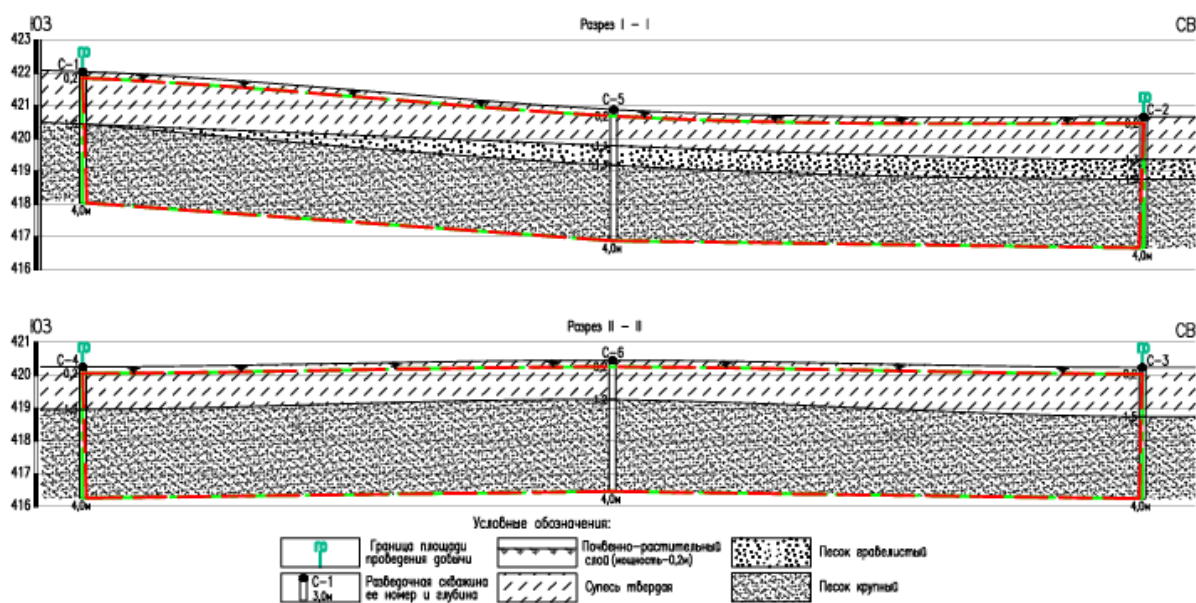
Рис. 2.7. Схема геологического строения участка «№9Ж».
