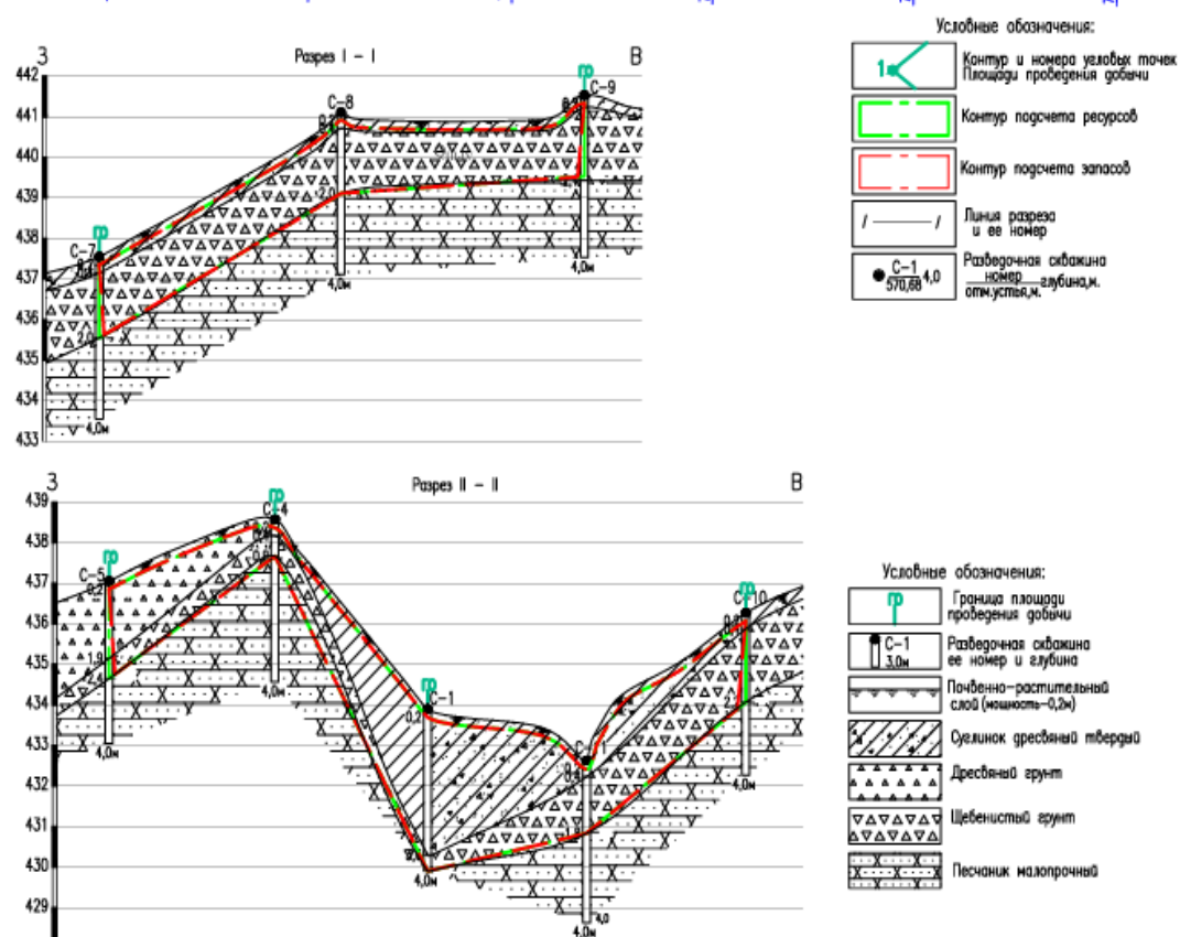
Рис. 2.8. Схема геологического строения участка «№4Д».
