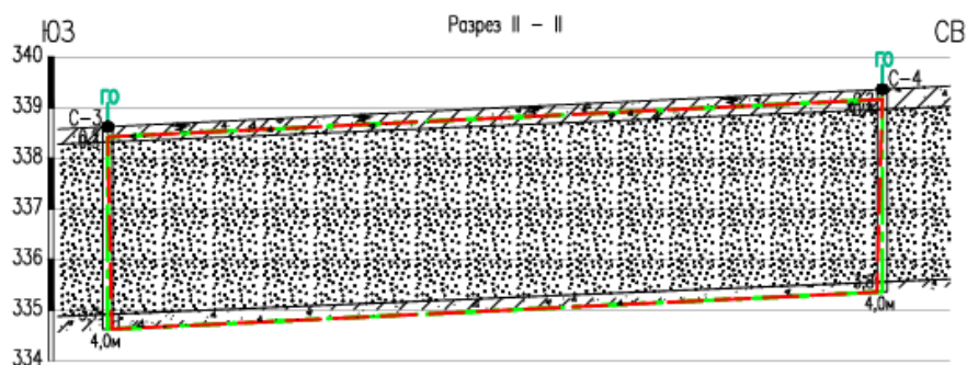
Рис. 2.16. Схема геологического строения участка «№28-Р».
