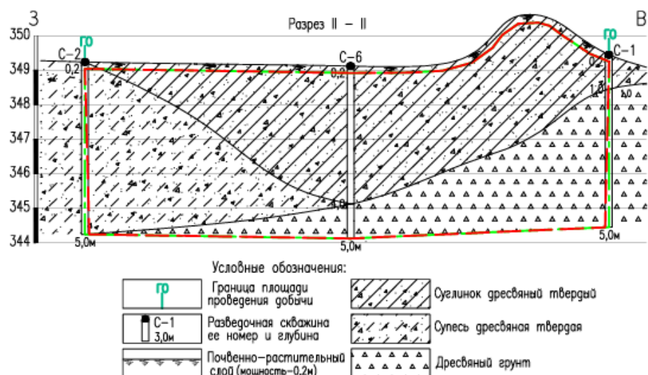
Рис. 2.14. Схема геологического строения участка «№7А».
