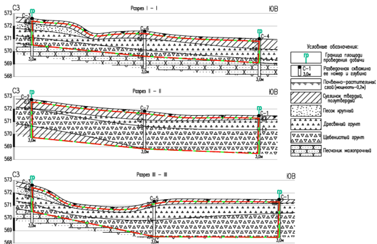
Рис. 2.5 Схема геологического строения участка «№1В»
