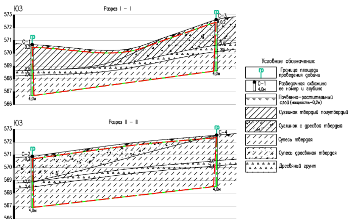
Рис. 2.6 Схема геологического строения участка «№1Г»
