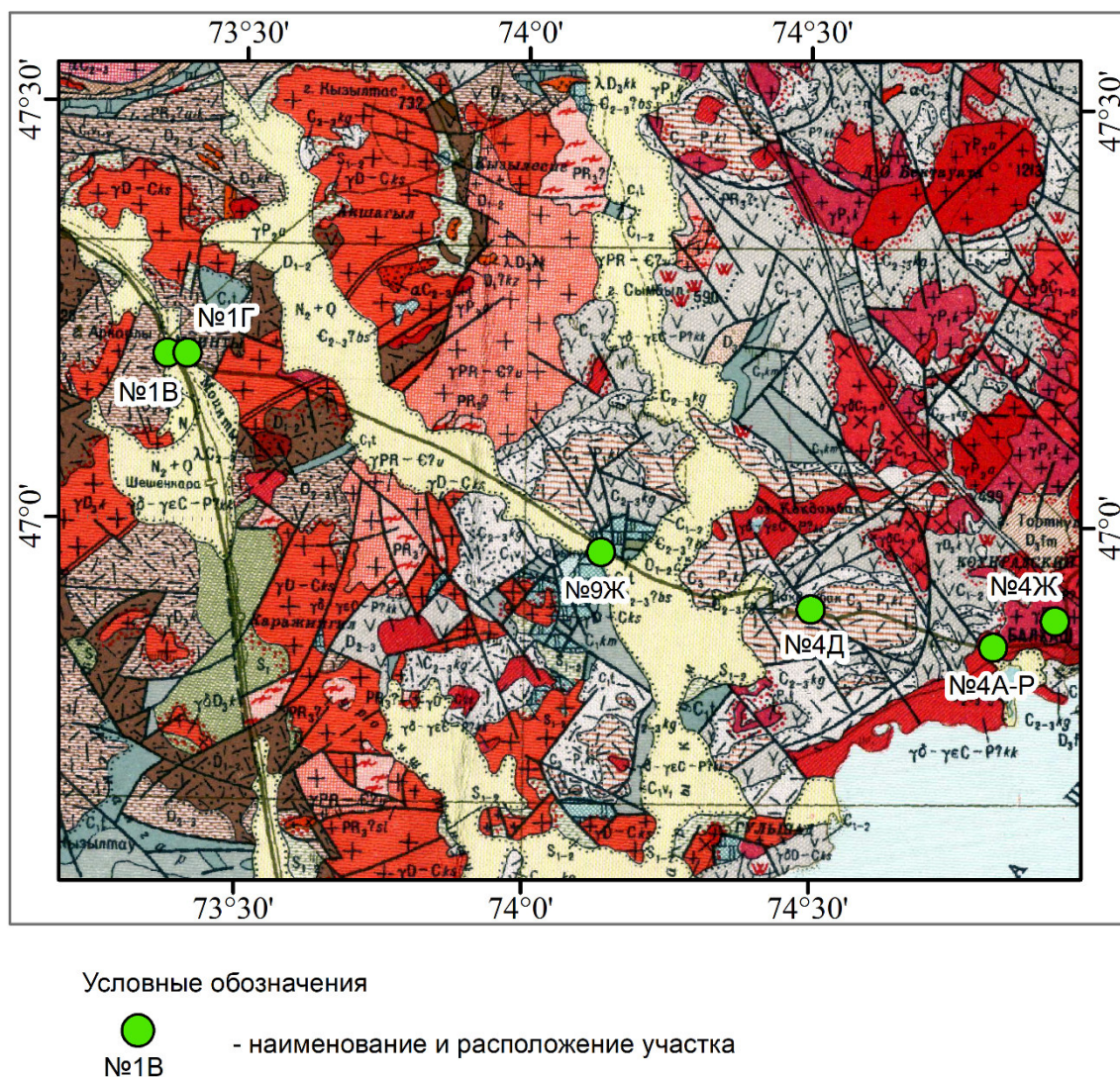
Рис.2.1 Геологическая карта расположения западной группы участков «№1В», «№1Г», «№9Ж», «№4Д», «№4А-Р». (выкопировка из геологической карты листа L-43. Масштаб 1:1 000 000)
