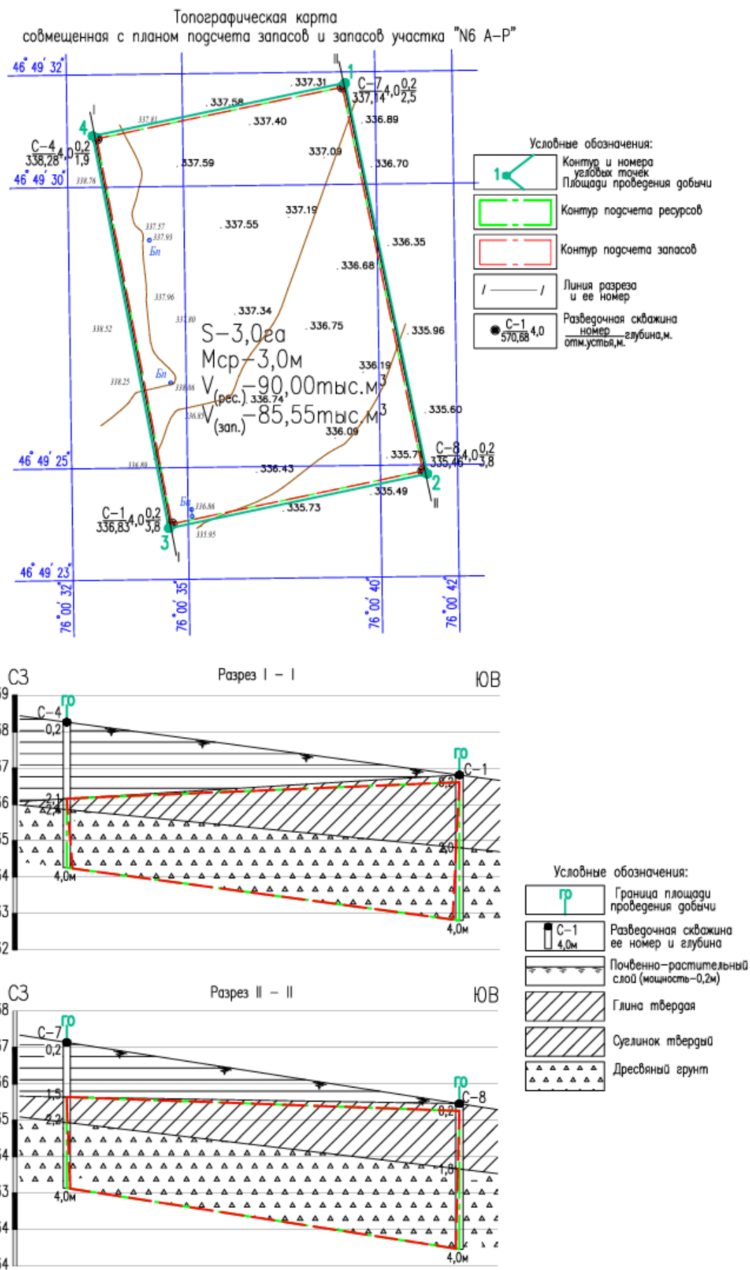
Рис. 2.13. Схема геологического строения участка «№6А-Р».
