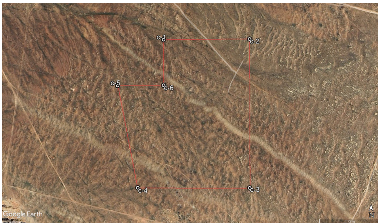
● c-1(1) местоположение и номер разведочной скважины, в скобках - угловые точки участка; - граница (контур) участка; - железная дорога Достык-Моинты Рис 1.9 Схема участка «№25-Р» с расположением скважин (на основе космоснимка)
