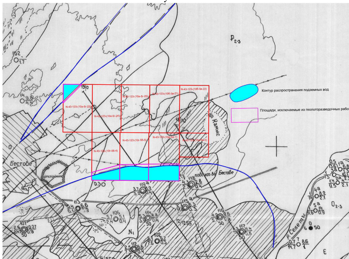
Контур распространения подземных вод и исключаемые площади Рисунок 2.2
