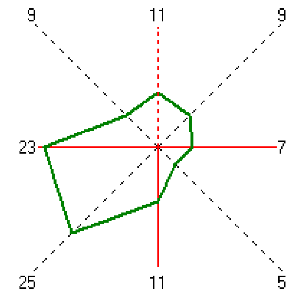
Рисунок 4.1 Роза ветров
