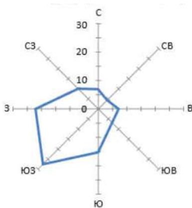
Рис. 1.2.5 Диаграмма повторяемости среднемноголетнего направления ветров, метеостанция Кокшетау (С-6,9%, СВ-4,4%, В-7,2%, ЮВ-6,9%, Ю-15,2%, ЮЗ-27,4%, З-22,2%, СЗ-10%).
