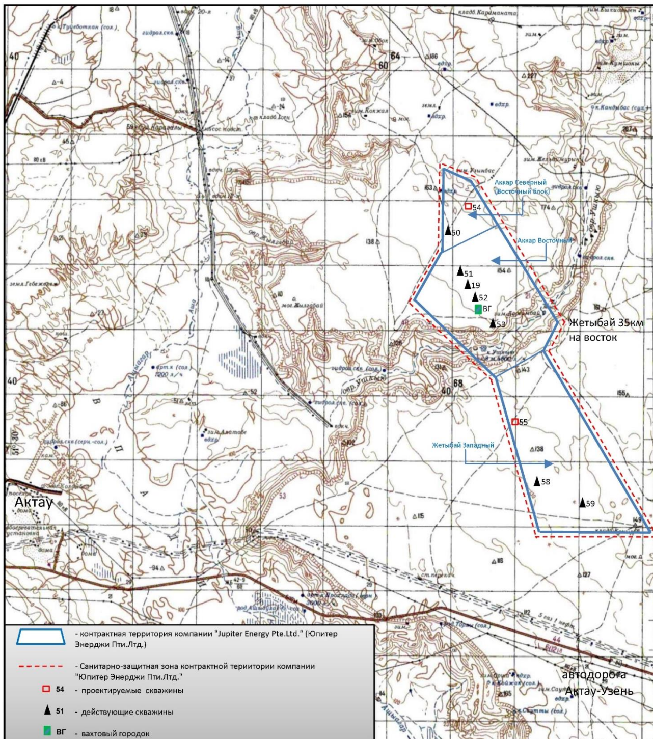
Рис. 2 Ситуационная карта расположения скважин на месторождении Аккар Восточный Компании «Jupiter Energy Pte. Ltd.»
