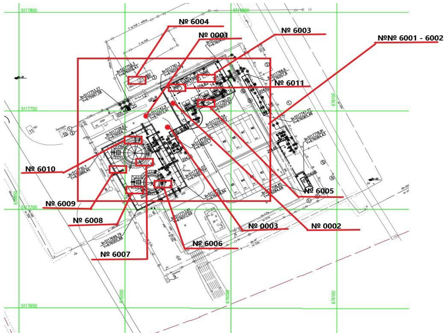
Карта-схема источников на период строительства
